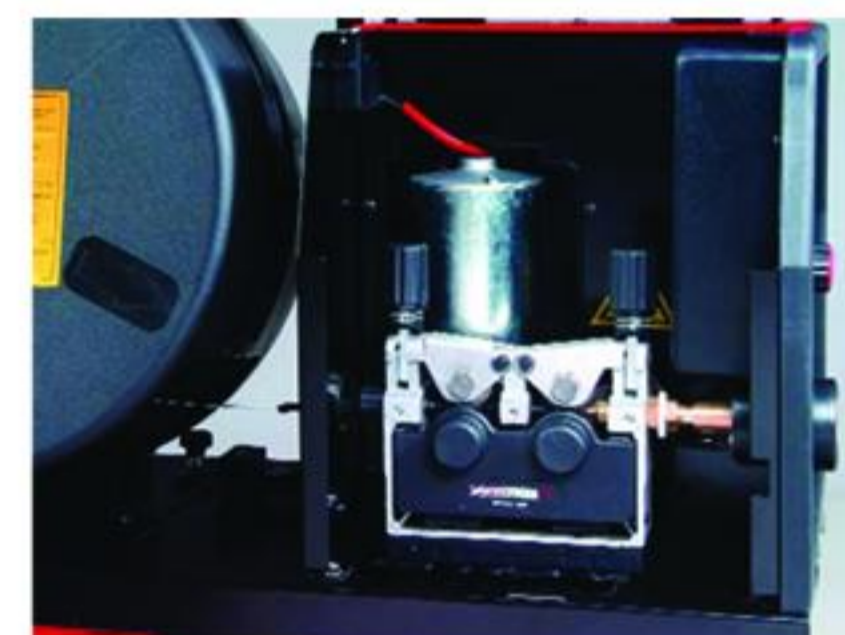
Τροφοδότης σύρματος 2 ή 4 ράουλα
